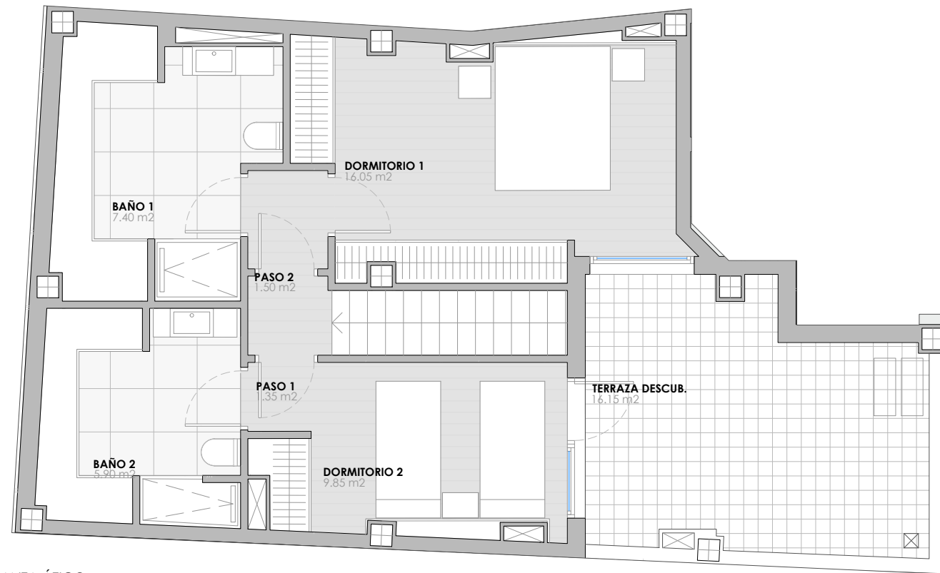
PLANTA ÁTICO
