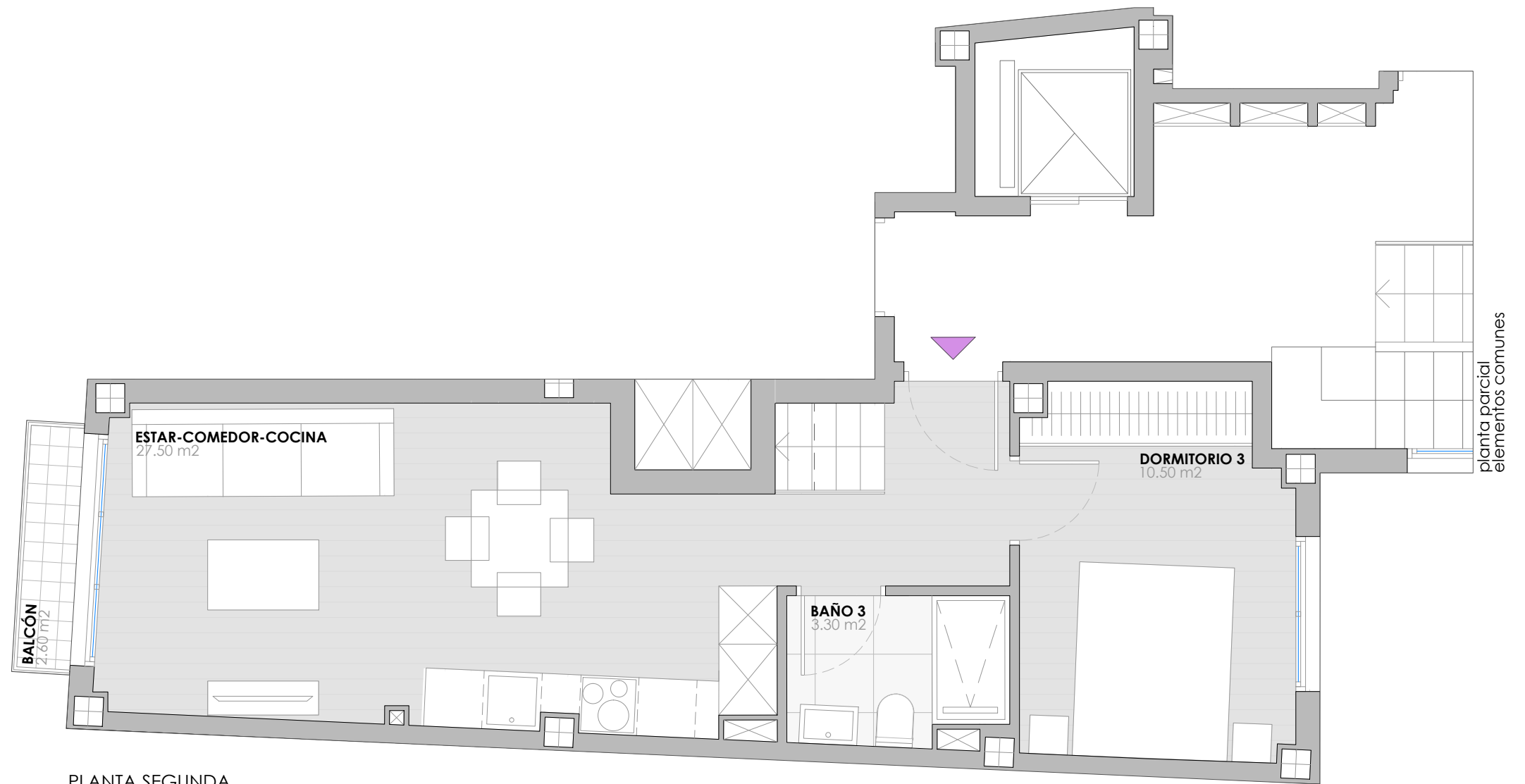
PLANTA SEGUNDA
